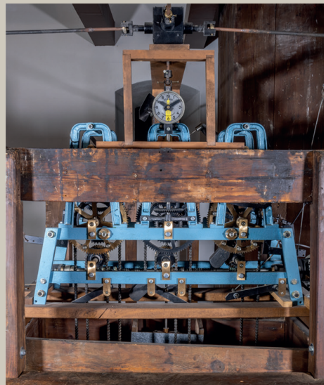
Současný hodinový stroj
