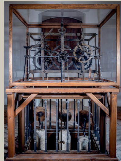
Barokní hodinový stroj
